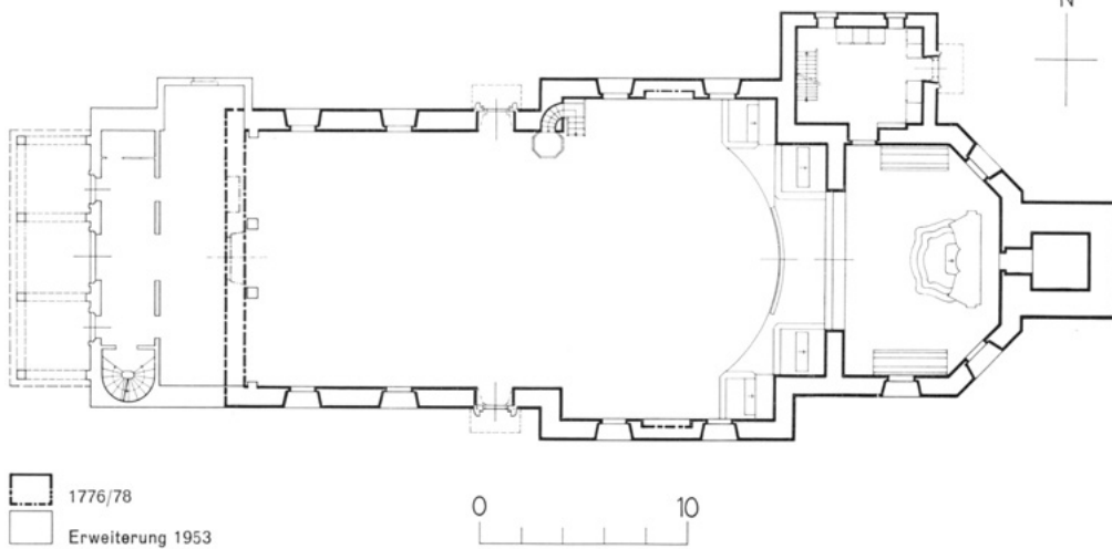
Abb. 185. Die Pfarrkirche zum Herzen Jesu in St. Fiden. Grundriß. Maßstab 1:400. – Text S. 196 f.
